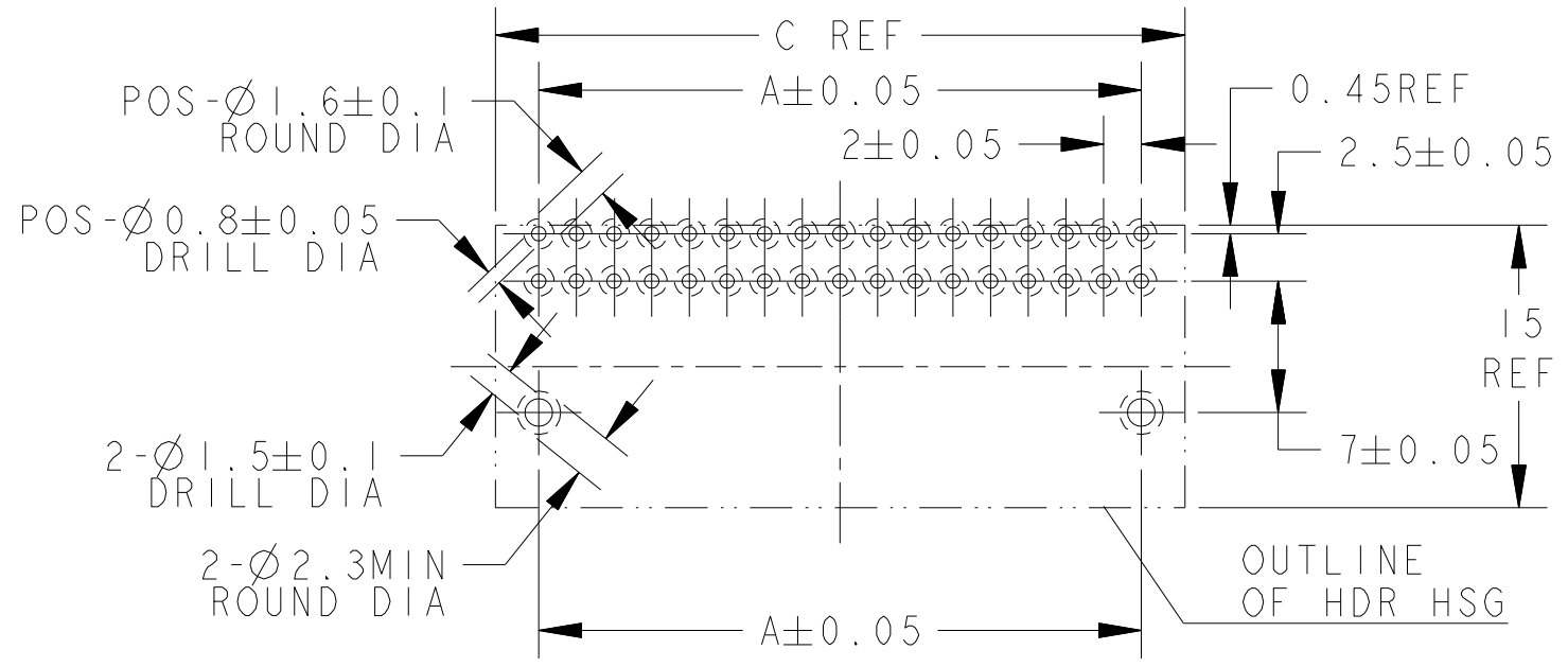
PCB板孔位尺寸示意图 PCB板厚度1.0~1.6MM±0.1
