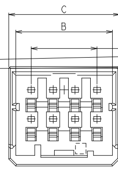
8POS(X-KEY):
